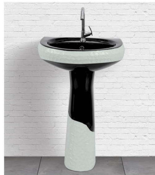
CLASSIC-002 L 570 W 445 H 845
